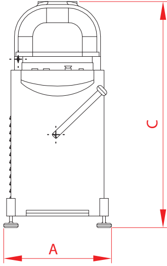
Ön Görünüş - Front View - вид спереди
